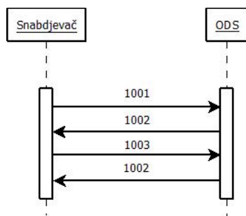
Slika 3: Sekvencijalni dijagram za proces Dostavljanje agregiranih podataka snabdjevaču
