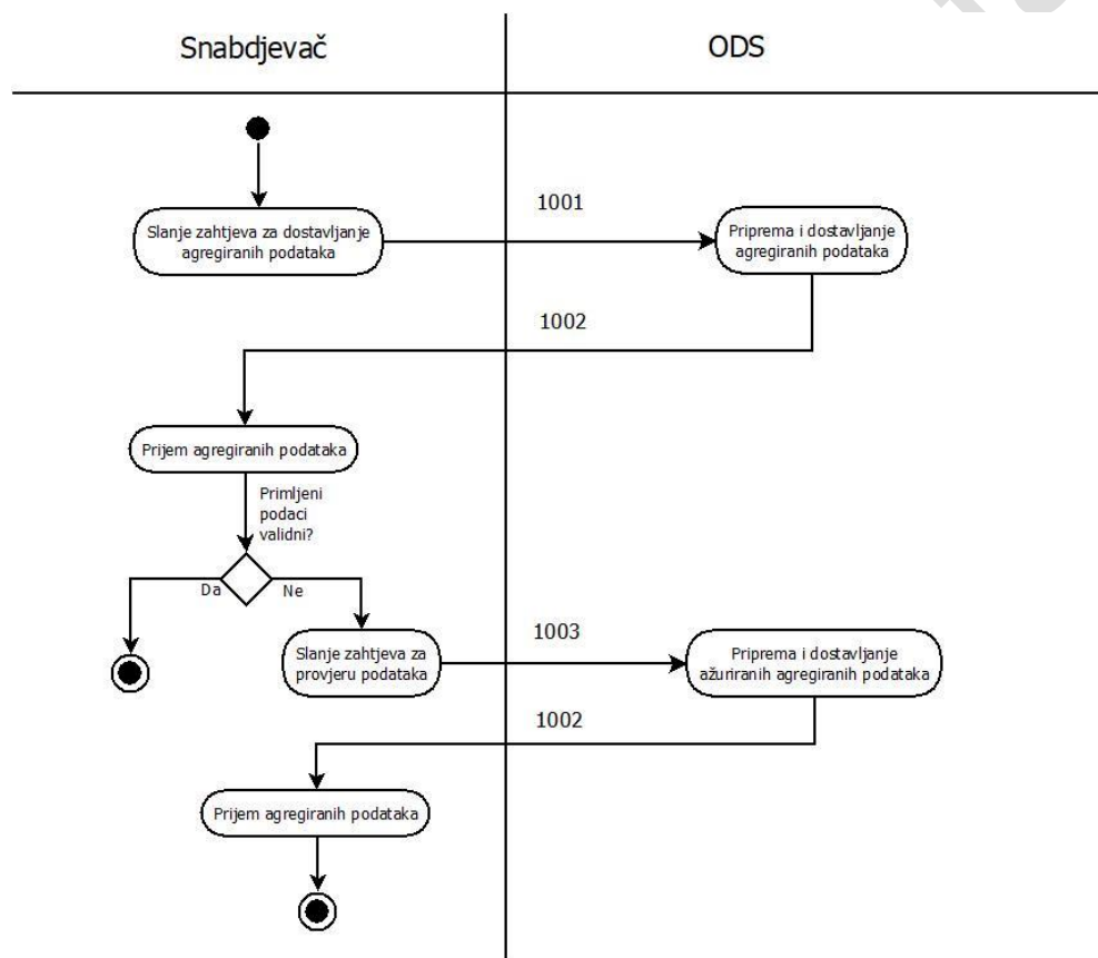
Slika 2: Dijagram aktivnosti procesa Dostavljanje agregiranih podataka snabdjevaču
